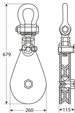
Dimensions in mm / Dimensiones en mm
