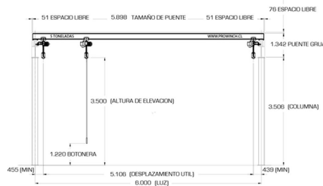
VISTA EN ELEVACION
