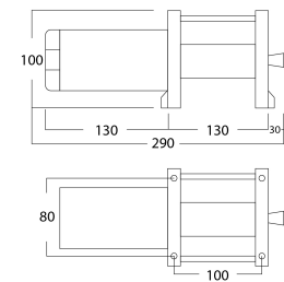
Dimensions in mm / Dimensiones en mm
