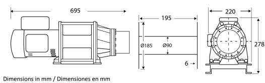
Dimensions in mm / Dimensiones en mm
